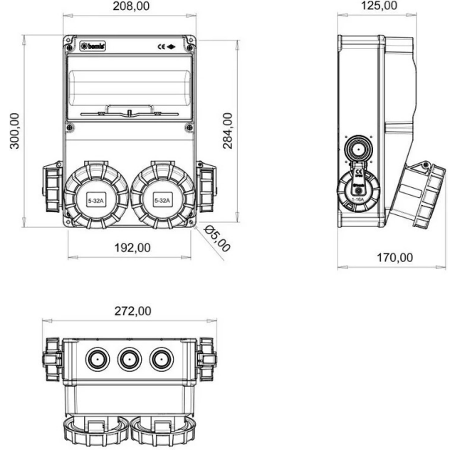
TEKNİK RESİM
