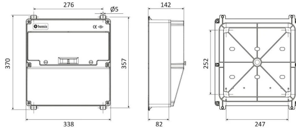
TEKNİK RESİM
