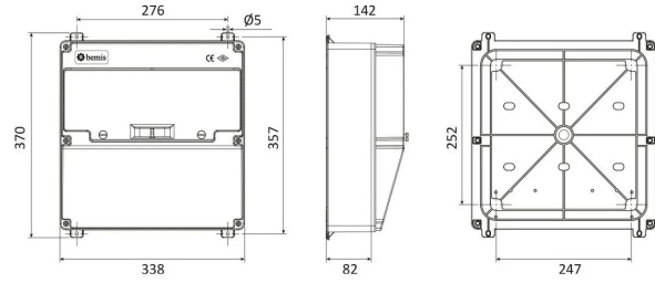
TEKNİK RESİM
