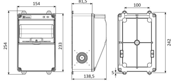
TEKNİK RESİM
