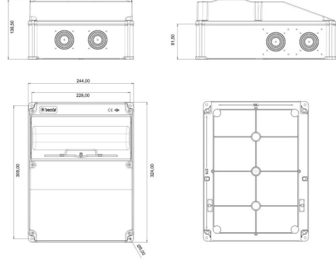
TEKNİK RESİM
