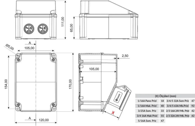
TEKNİK RESİM
