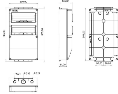
TEKNİK RESİM
