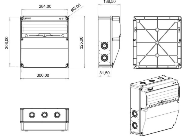
TEKNİK RESİM
