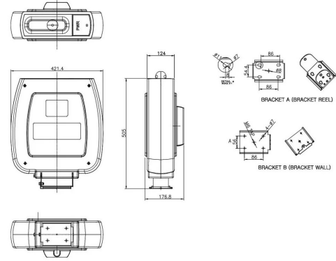
TEKNİK RESİM
