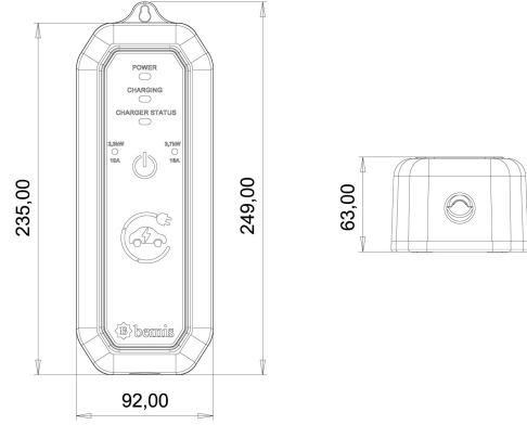
TEKNİK RESİM
