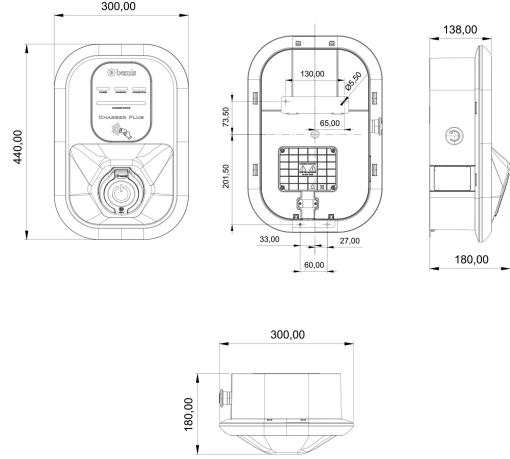
TEKNİK RESİM
