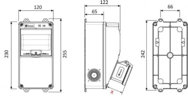
(X) Ölçüleri / Dimensions (mm)
