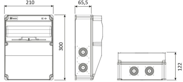
TEKNİK RESİM
