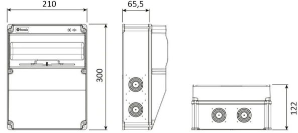
TEKNİK RESİM
