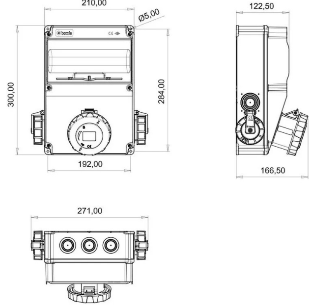
TEKNİK RESİM
