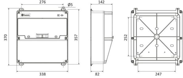
TEKNİK RESİM
