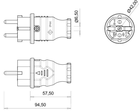
TEKNİK RESİM
