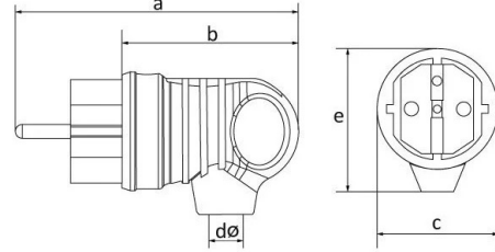
Ölçüler / Dimensions (mm)
