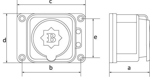
Ölçüler / Dimensions (mm)
