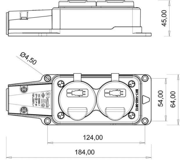
TEKNİK RESİM
