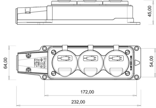
TEKNİK RESİM
