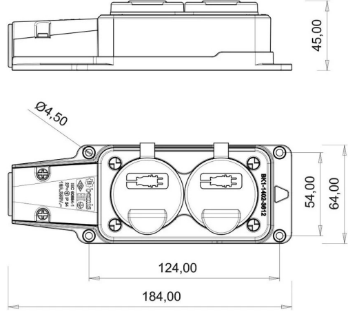
TEKNİK RESİM
