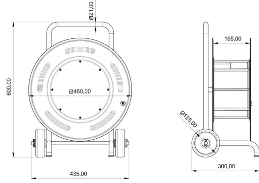
TEKNİK RESİM
