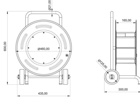
TEKNİK RESİM
