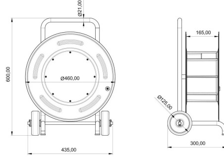
TEKNİK RESİM
