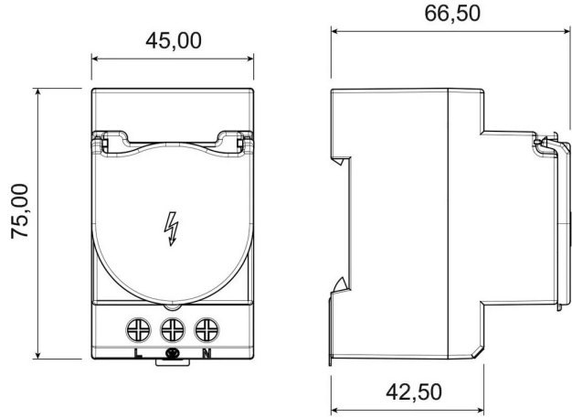
TEKNİK RESİM
