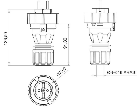
TEKNİK RESİM
