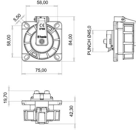
TEKNİK RESİM
