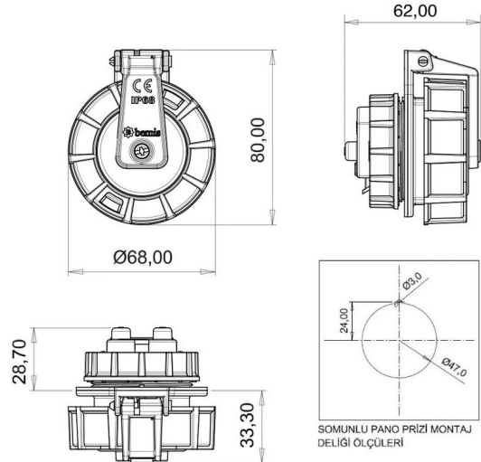
TEKNİK RESİM
