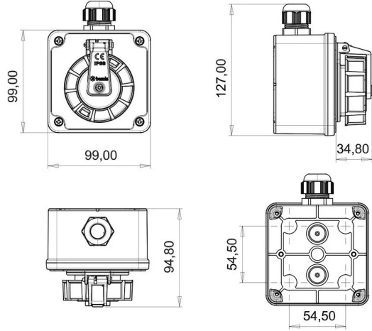
TEKNİK RESİM
