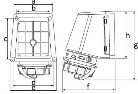
Ölçüler / Dimensions (mm)
