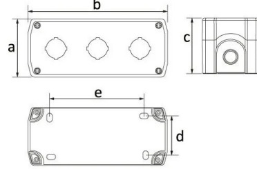
Ölçüler / Dimensions (mm)
