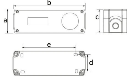
Ölçüler / Dimensions (mm)
