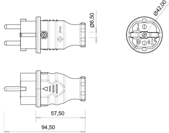
TEKNİK RESİM
