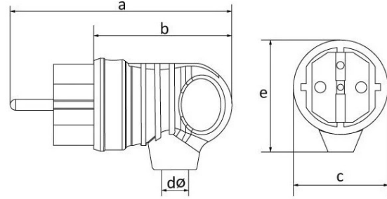
TEKNİK RESİM
