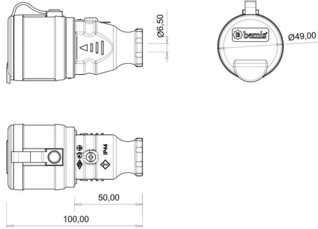
TEKNİK RESİM
