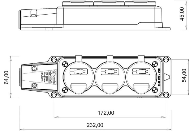
TEKNİK RESİM
