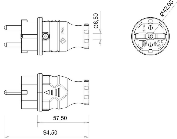
TEKNİK RESİM
