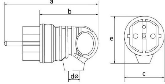
TEKNİK RESİM
