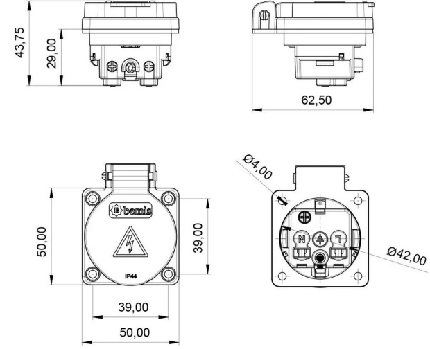
TEKNİK RESİM
