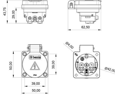
TEKNİK RESİM
