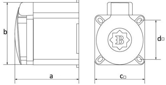
Ölçüler / Dimensions (mm)
