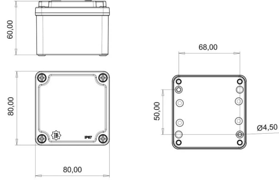
TEKNİK RESİM
