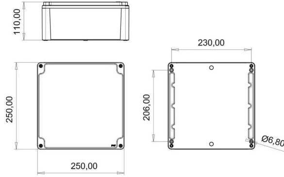
TEKNİK RESİM
