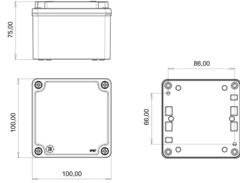
TEKNİK RESİM
