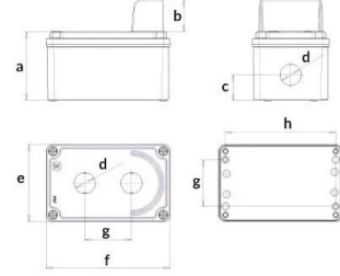
Ölçüler / Dimensions (mm)
